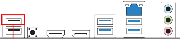
USB BIOS 플래시백 포트
